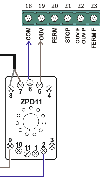
Détecteur de boucle LDP1 - 230v
